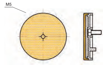
Catadióptrico redondo (Ø55). Catadióptrico redondo (Ø55).
