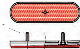
Catadióptrico ovalado (96x27). Trasero. Catadióptrico ovalado (96x27). Traseiro.
