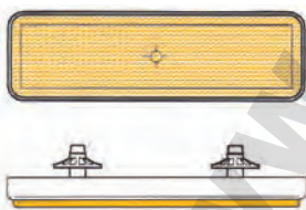
Catadióptrico rectangular (91x25). Lateral. Catadióptrico rectangular (91x25). Lateral.
