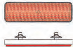
Catadióptrico rectangular (91x25). Trasero. Catadióptrico rectangular (91x25). Traseiro.
