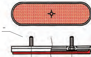
Catadióptrico ovalado (96x27). Trasero. Catadióptrico ovalado (96x27). Traseiro.
