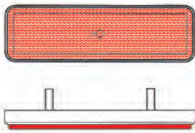
Catadióptrico rectangular (91x25). Trasero Catadióptrico rectangular (91x25). Traseiro
